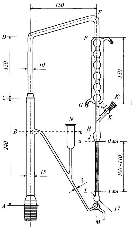
Рисунок 2.8.12.-1. Прилад для визначення вмісту ефірних олій у рослинних лікарських засобах Розміри зазначені у міліметрах
