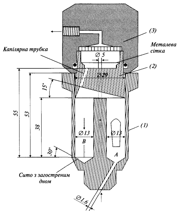
Рисунок 2.9.3.-6. Проточна кювета Розміри зазначені у міліметрах
