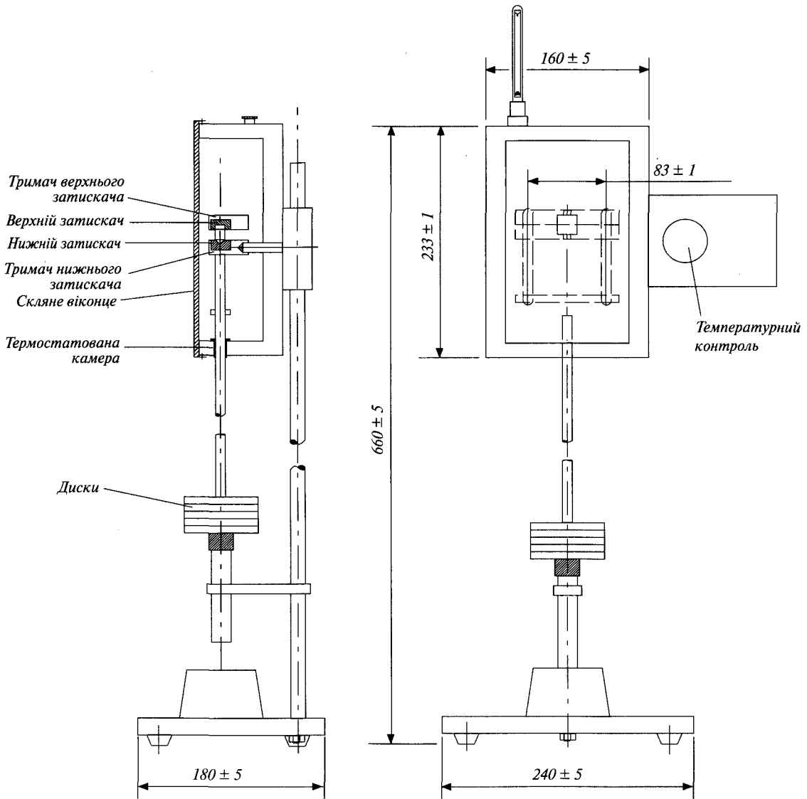
Рисунок. 2.9.24-1. Прилад для визначення стійкості супозиторіїв і несаріїв до руйнування Розміри зазначені в міліметрах
