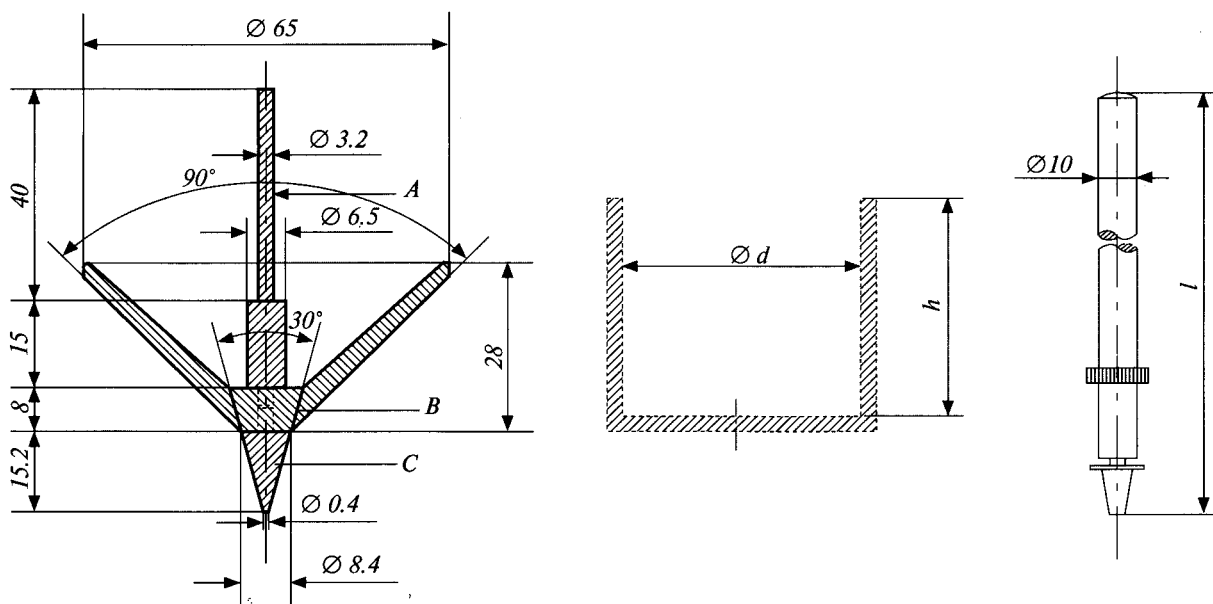
Рисунок 2.9.9.-2. Конус ( m=102.5 г), підходящий контейнер ( d=102 мм або 75 мм, h \geq 62 мм) і стрижень ( l=162 мм; m=47.5 г). Розміри зазначені в міліметрах
