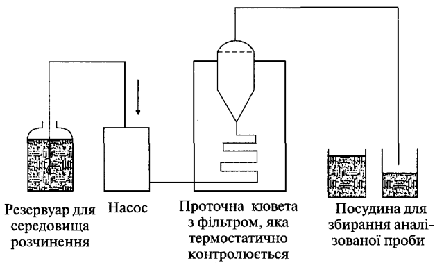
Рисунок 2.9.3.-3. Проточний прилад
