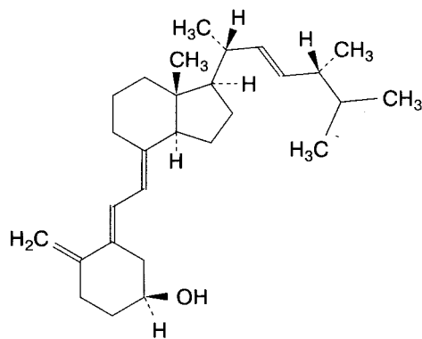
А. (5 E ,7 E ,22 E )-9,10-секоергоста-5,7,10(19),22-тетраен-3β-ол ( транс -вітамін D 2 ),
