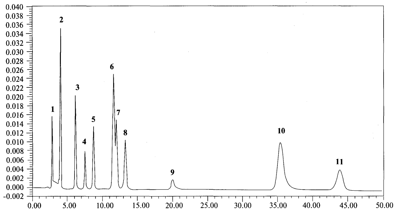
Рисунок 0049.-1. Хроматограма, одержана при визначенні супровідних домішок: піки парацетамолу та домішок
