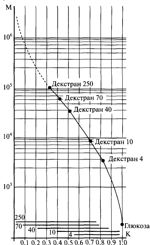
Рис. 2.2.39.-1. Приклад калібрувальної кривої. Пунктиром позначена частина калібрувальної кривої, одержана екстраполюванням. Горизонтальними лініями в нижній частині рисунка позначені ширини i положення хроматографічних ліній, одержаних для кожного декстрану для калібрування
