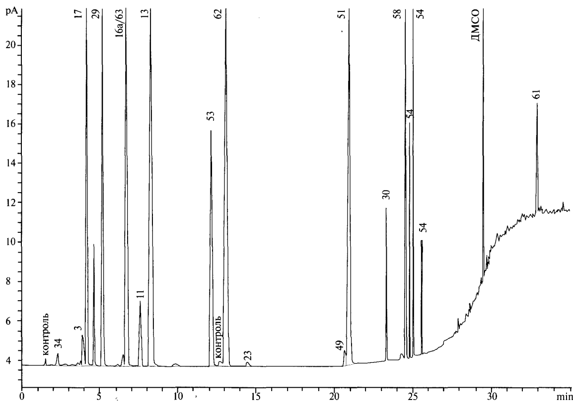
Рисунок 2.4.24.-2. Хроматограма залишкових розчинників класу 2 в умовах, описаних для системи А і пробопідготовки 1. Полуменево-іонізаційний детектор.
