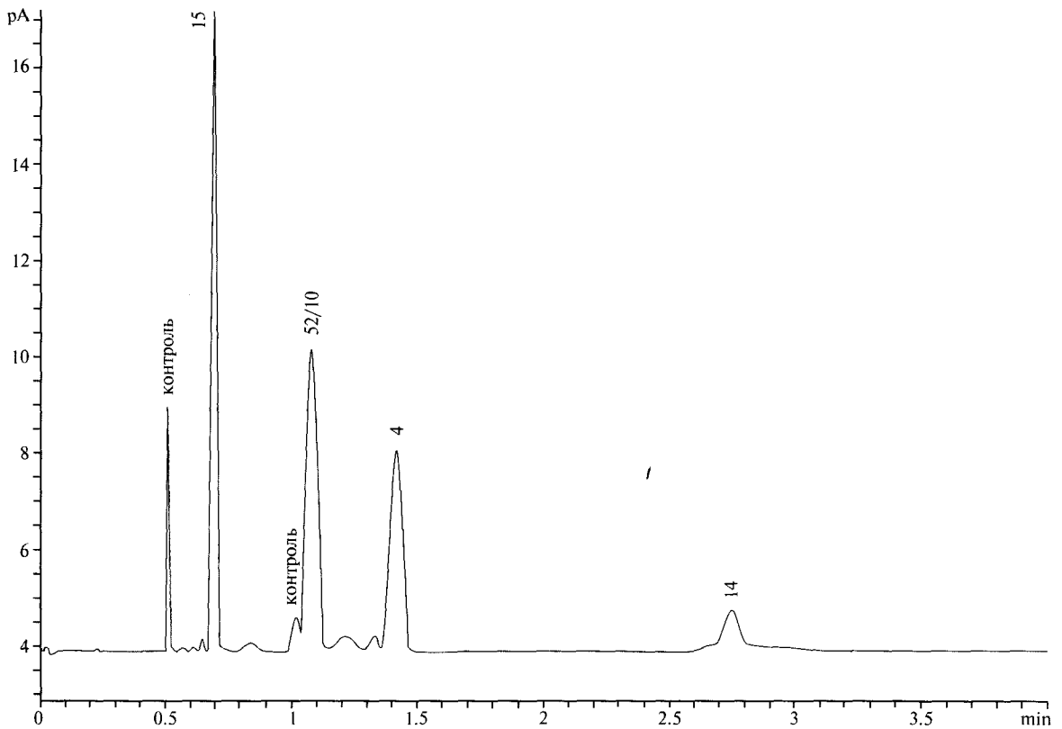
Рисунок 2.4.24.-3. Хроматограма залишкових розчинників класу 1 в умовах, описаних для системи В і прободготовки 1. Полуменево-іонізаційний детектор.
