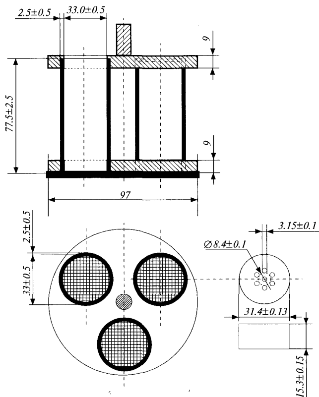
Рисунок 2.9.1.-2. Обладнання В Розміри зазначені у міліметрах
