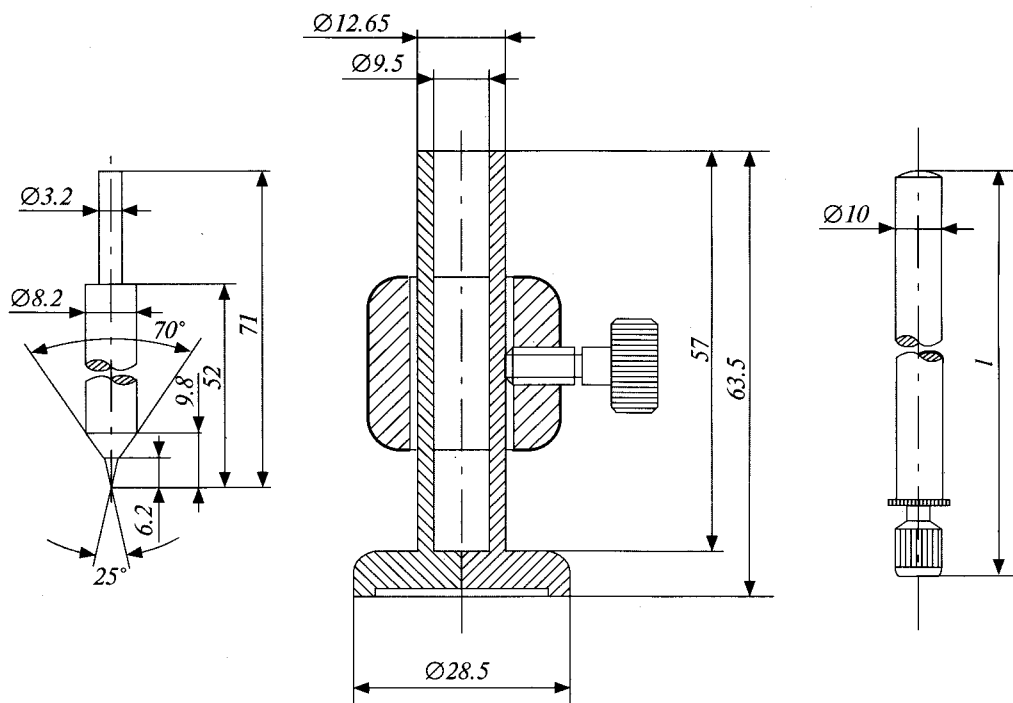
Рисунок 2.9.9.-3. Мікроконус ( m=7.0 г), підхожий контейнер і стрижень ( l=116 мм; m=16.8 г) Розміри зазначені в міліметрах
