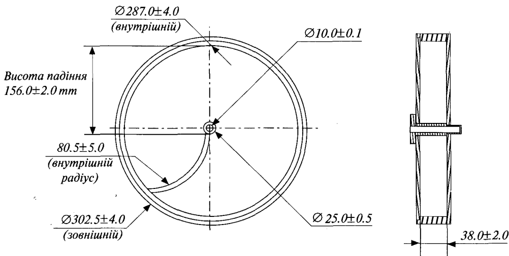
Рисунок 2.9.7.-1. Прилад для визначення стираності таблеток Розміри зазначені у міліметрах
