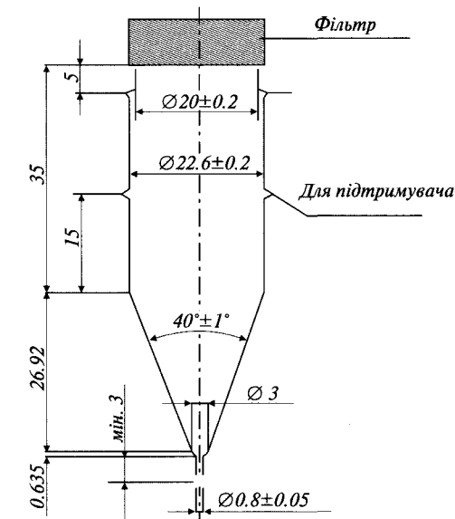
Рисунок 2.9.3.-3. Проточний прилад
