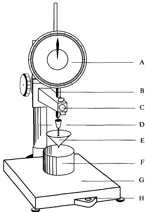
Рисунок 2.9.9.-1. Пенетрометр
