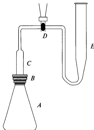
Рисунок 3.2.1.-2. Прилад для визначення арсену
