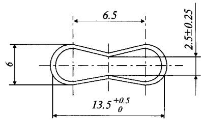
Підтримувач для 12.0 мм кювети
