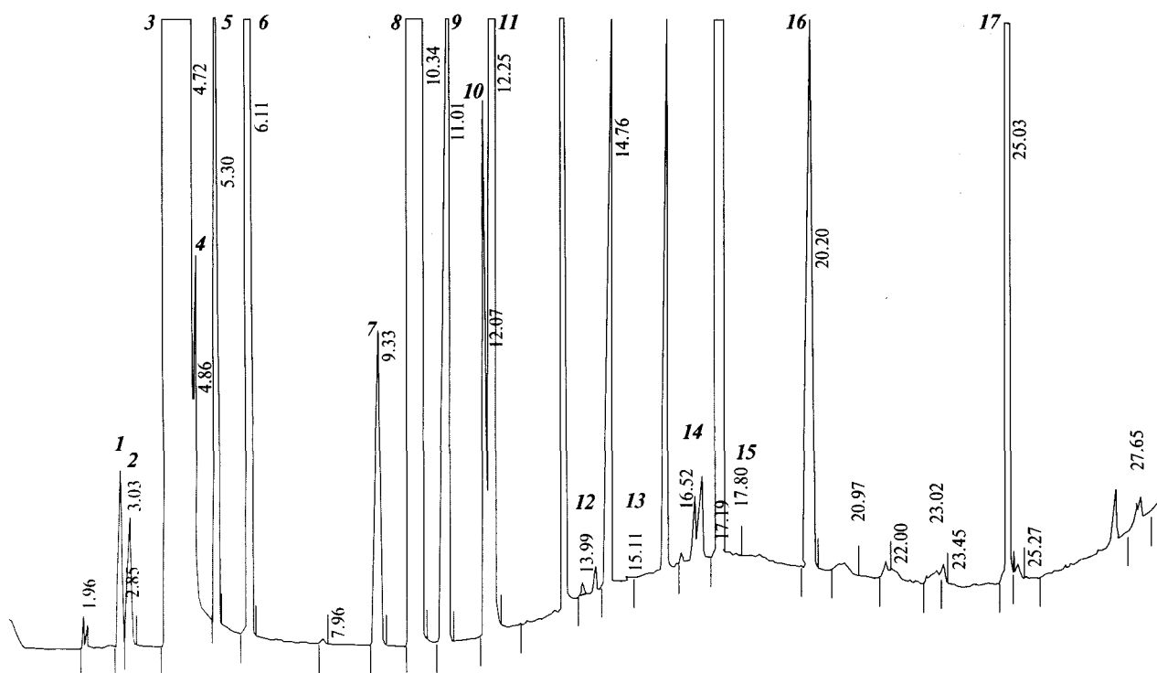
Рисунок 1317.-1. Летки домішки: типова хроматограма суміші етанолу і шістнадцяти домішок
