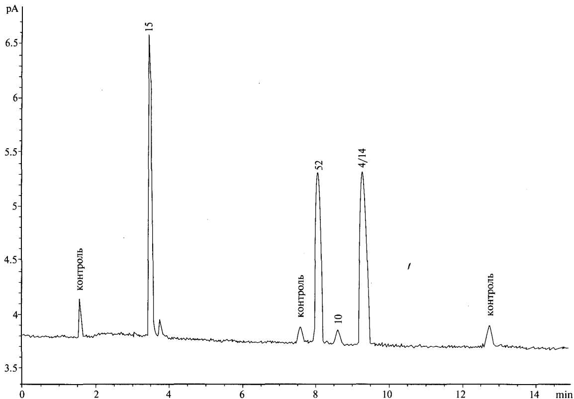
Рисунок 2.4.24.-1. Типова хроматограма залишкових розчинників класу 1 в умовах, описаних для системи А та пробопідготовки 1. Полуменево-іонізаційний детектор.
