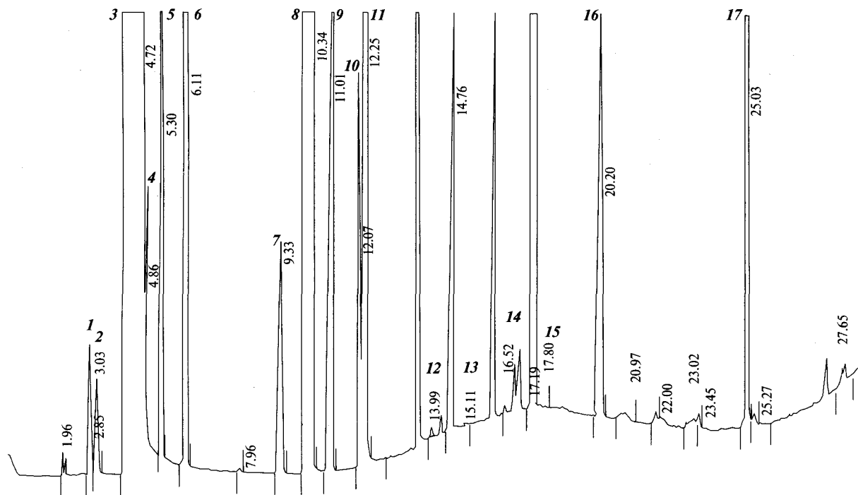
Рисунок 1318.-1. Леткі домішки: типова хроматограма суміші етанолу і шістнадцяти домішок
