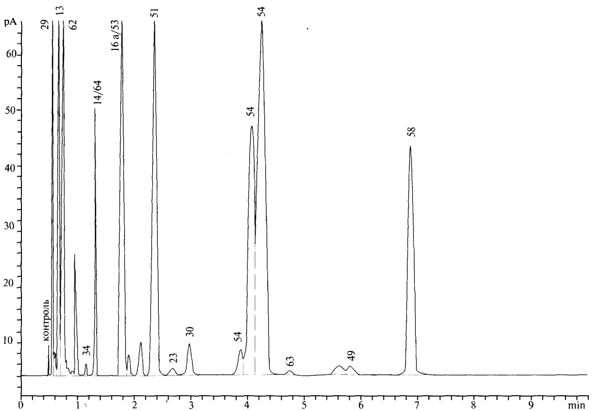
Рисунок 2.4.24.-4. Хроматограма залишкових розчинників класу 2 в умовах, описаних для системи В і прободготовки 1. Полуменево-іонізаційний детектор.
