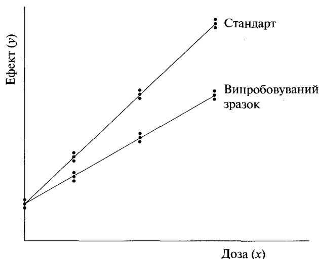
Рисунок 3.3.1.-1. Модель кутових коефіцієнтів для кількісного визначення 2 \times 3 + 1
