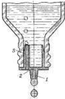
Рис. 5. Крапельниця з центральним краплеутворенням ЛНПО «Прогрес»:
