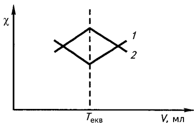
Рис. 3.14. Криві високочастотного титрування
