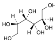
B. D-idoitol,
