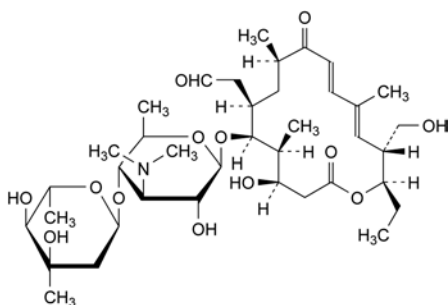
A. desmynosyltylosin,
