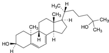
A. 9β,10α-cholesta-5,7-diene-3β,25-diol,
