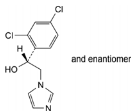
A. (RS)-1-(2,4-dichlorophenyl)-2-(1H-imidazol-1-yl)ethanol,
