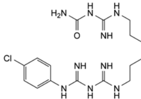
B. [[6-[[[(4-chlorophenyl)carbamimidoyl]carbamimidoyl]amino]hexyl]carbamimidoyl]urea,
