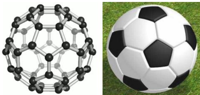
Рис. 6. Модель фулерену C_{60} та фотографія футбольного м'яча
