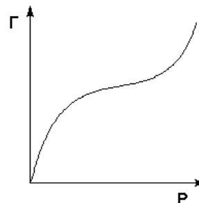
Рис. 6. Ізотерма полімолекулярної адсорбції
