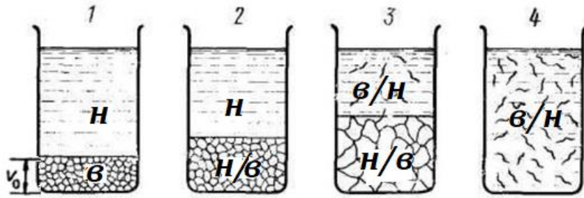
Рис. 2. Етапи набухання ( н – молекули НМР; в – молекули ВМР)
