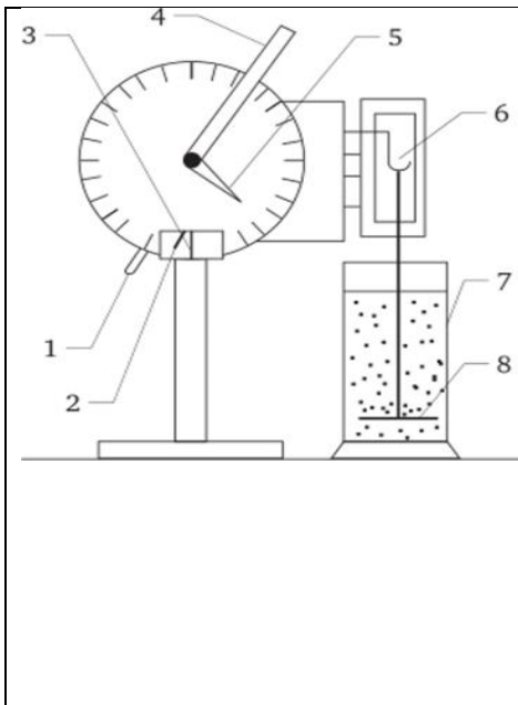
Рис. 5. Схема седиментометру на базі торсійних вагів:
