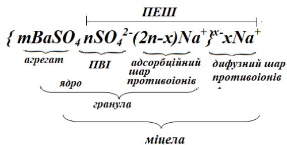
Будова частки ліофобного золю при надлишку Na_2SO_4
