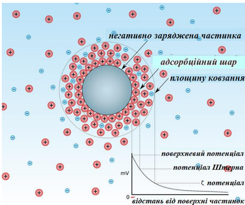
Будова подвійного електричного шару
