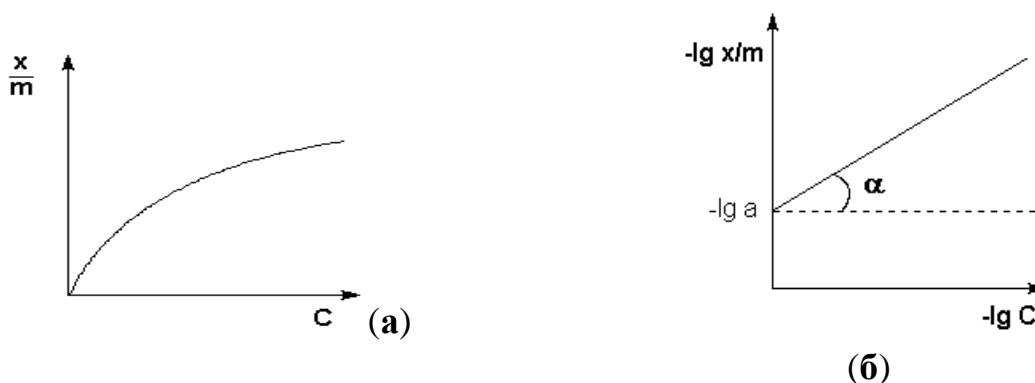
Ізотерма адсорбції Фрейндліха у звичайних (а) і логарифмічних (б) координатах
