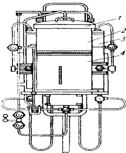
Рис. 2 Схема апарата для одержання апірогенної води ЦАНДІ
