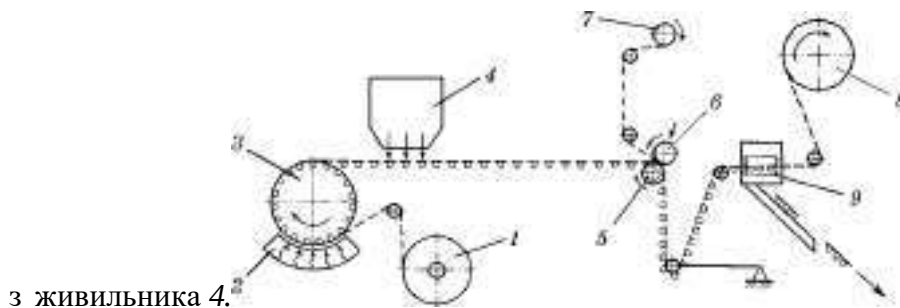
Рис. 1. Схема автомата безперервного формування
