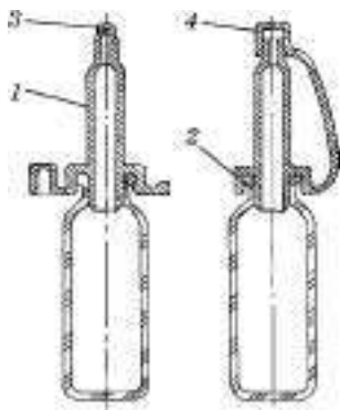
Рис. 7. Поршневий дозатор для об'ємного дозування: 1 — пробка з отвором для поршня; 2 — висувний поршень-дозатор; 3 — насадка з випускним отвором; 4 — герметизаційна кришка. При великій дозі доцільно застосовувати об'ємні дозувальні засоби, що зазвичай додаються
