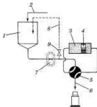
Рис.4. Схема роботи дозатора автомата (модель 3061):
