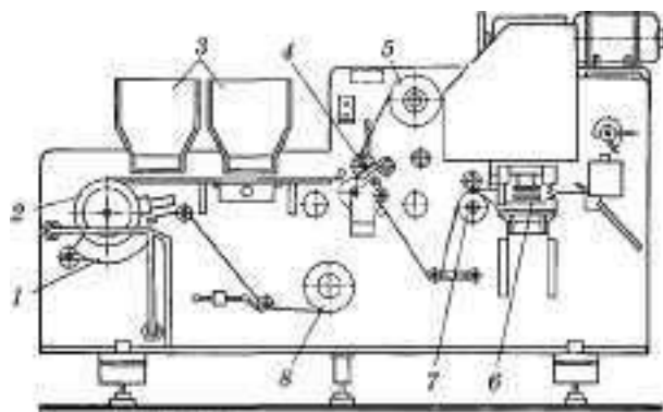
Рис. 12. Автомат для маркування й упаковки ампул місткістю 1 мл:
