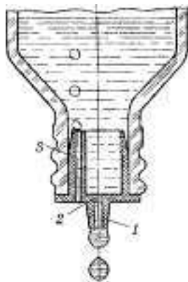
Рис. 5. Крапельниця з центральним краплеутворенням ЛНПО «Прогрес»: 1 — краплеутворювальна трубка; 2 — отвір для витікання рідини; 3 — повітряний канал
