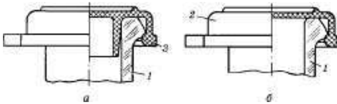
Рис. 8. Закупорка натягувальною кришкою:
