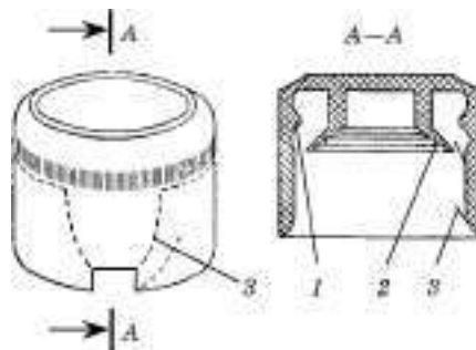
Рис. 9. Пробка з контролем першого розкриття: 1 — виступ для утримання пробки; 2 — конічна гофрована частина, що відгинається; 3 — надрізи для полегшення розкриття
