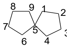
спіро [4,4] нонан
