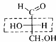
L-гліцериновий альдегід
