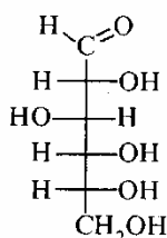
D-глюкоза
