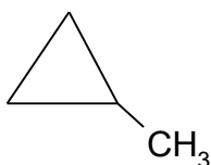
Метилциклопропан
