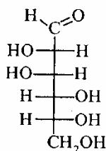
D-манноза
