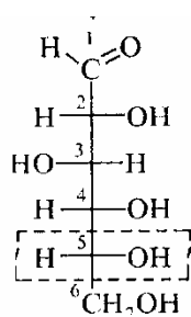
D-глюкоза
