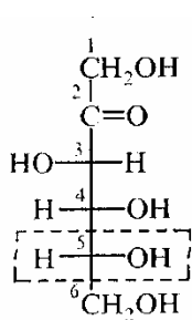
D-фруктоза
