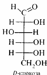
D-глюкоза
