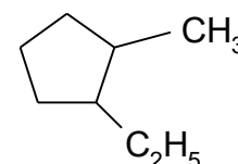
1-метил-2-етилциклопентан
