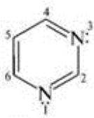
1,3-діазин
