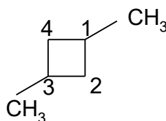
1,3-диметилциклобутан
