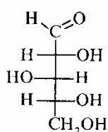
D-ксилуза
