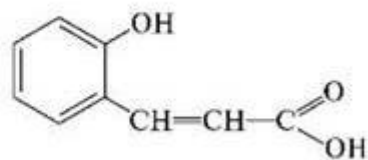
2-гідроксикорична к-та
