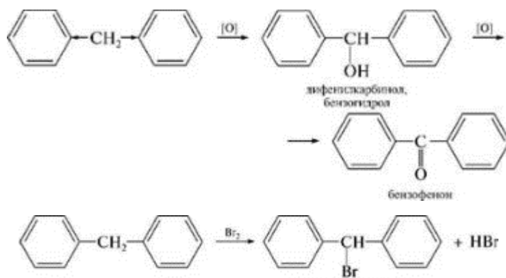
дифенілбромметан
