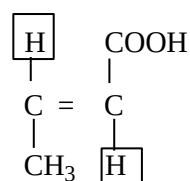
Транс-кротонова к-та
