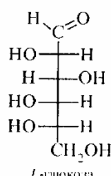
L-глюкоза
