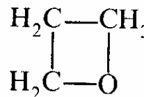
оксетан
