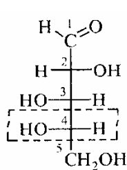
L-арабіноза
