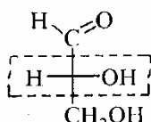
D-гліцериновий альдегід
