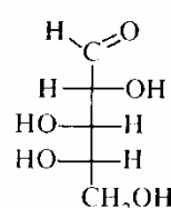
L-арабіноза
