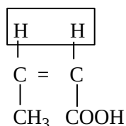
Цис-кротонова к-та
