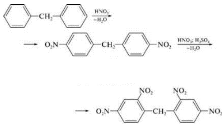
2,4,2,4' -тетранітродифенілметан
