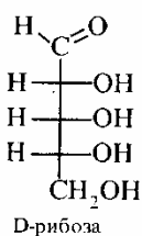
D-рибоза
