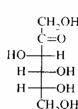
D-фруктоза
