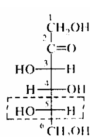
L-сорбоза
