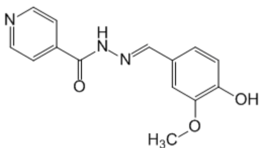
Фтівазид
