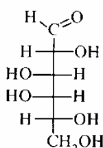
D-галактоза
