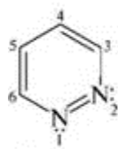
1,2-діазин
