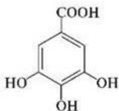
Галова к-та
