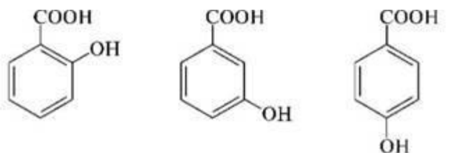
м-гідроксибензойна к-та
