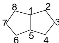
біцикло [3,3,0]октан
