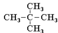
2,2-диметилпропан
