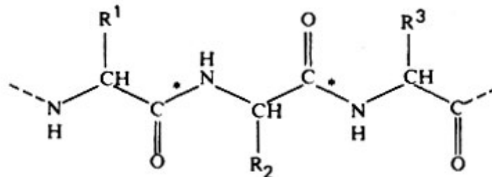
Схема 3. Частина молекули поліпептиду, утворена трьома залишками амінокислоти. Пептидні зв'язку позначені зірочкою
