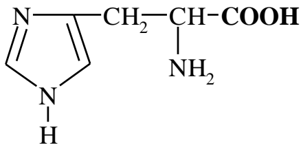
Гістидин
