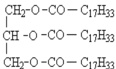
триоленоілгліцерин
