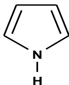
пірол
