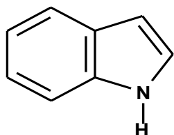
індол
