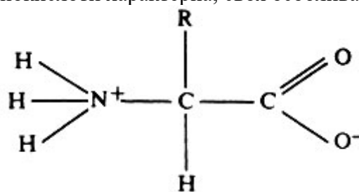
Рисунок. 1. Нейтральна цвіттеріонна форма амінокислоти (-NH 2 , основна група, має сильну схожість до Н + - іонів) (-COOH, кислотна група, дисоціює з вивільненням Н + -іонів).
