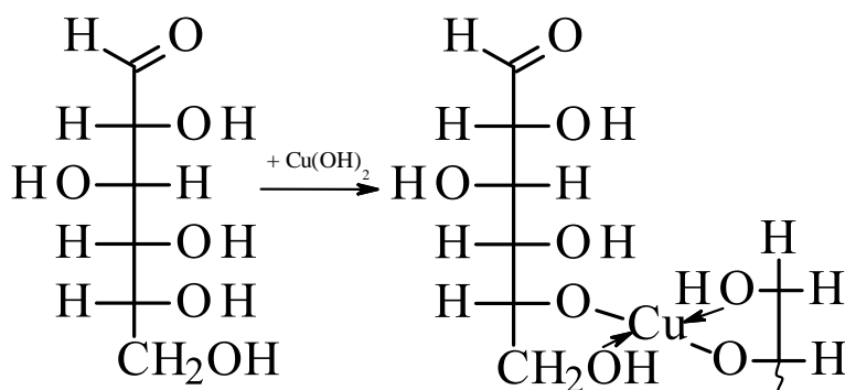
D-глюкоза
