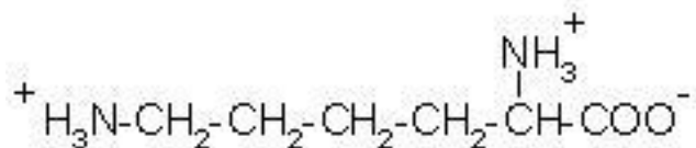
Лізин
