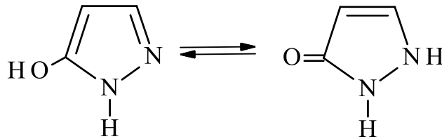
Піразолон-5
