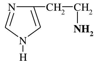
Гістамін
