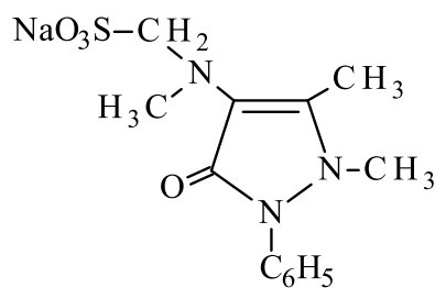
Амідопірін
