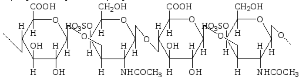
Фрагмент хондроїтин-4-сульфату
