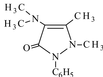
Піразолон-5
