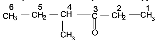
4 - метилгексанон - 3
