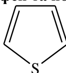
тіофен
