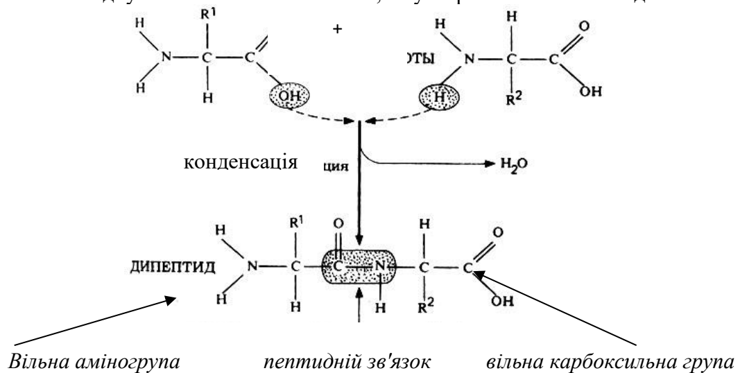
Схема. 2. Утворення дипептиду в результаті конденсації двох амінокислот
